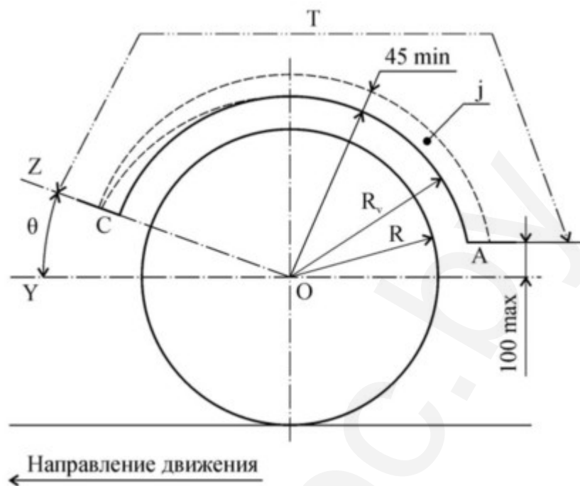
б) Расположение брызговика и энергопоглощающего устройства
