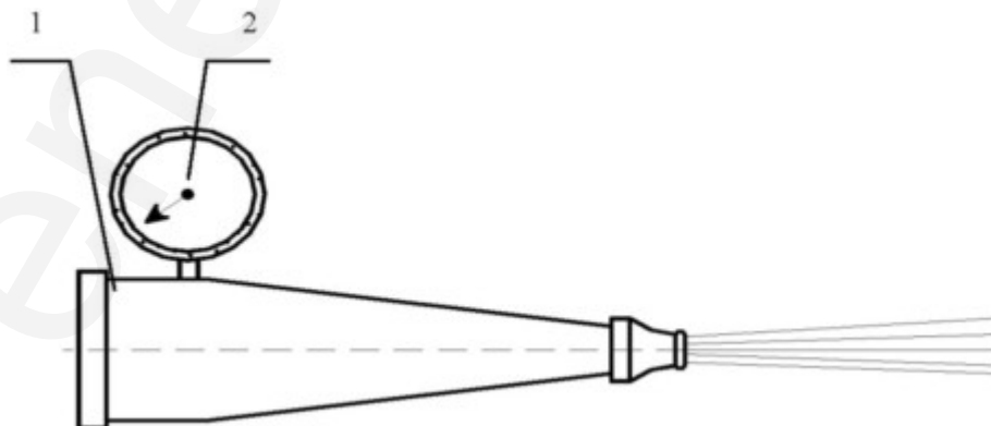
Схема ствола-водомера
