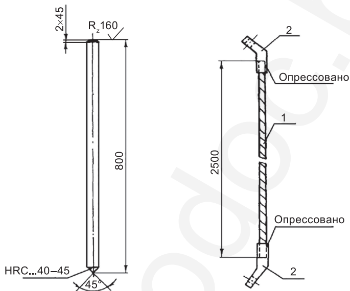
Заземлитель
