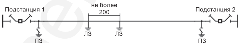
Рисунок К.5 – ВЛ 6–20 кВ разземлена в РУ и заземлена на линейные заземления, установленные с обеих сторон от места работы
