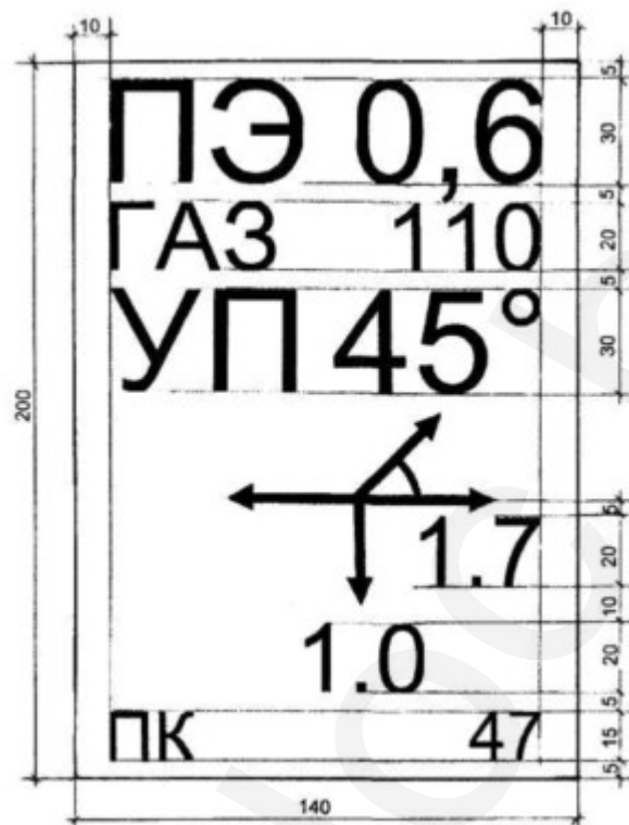
Рисунок 3. Полиэтиленовый газопровод, диаметр – 110 мм, угол поворота – 45°.
